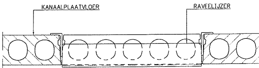
DRSN. A-A
