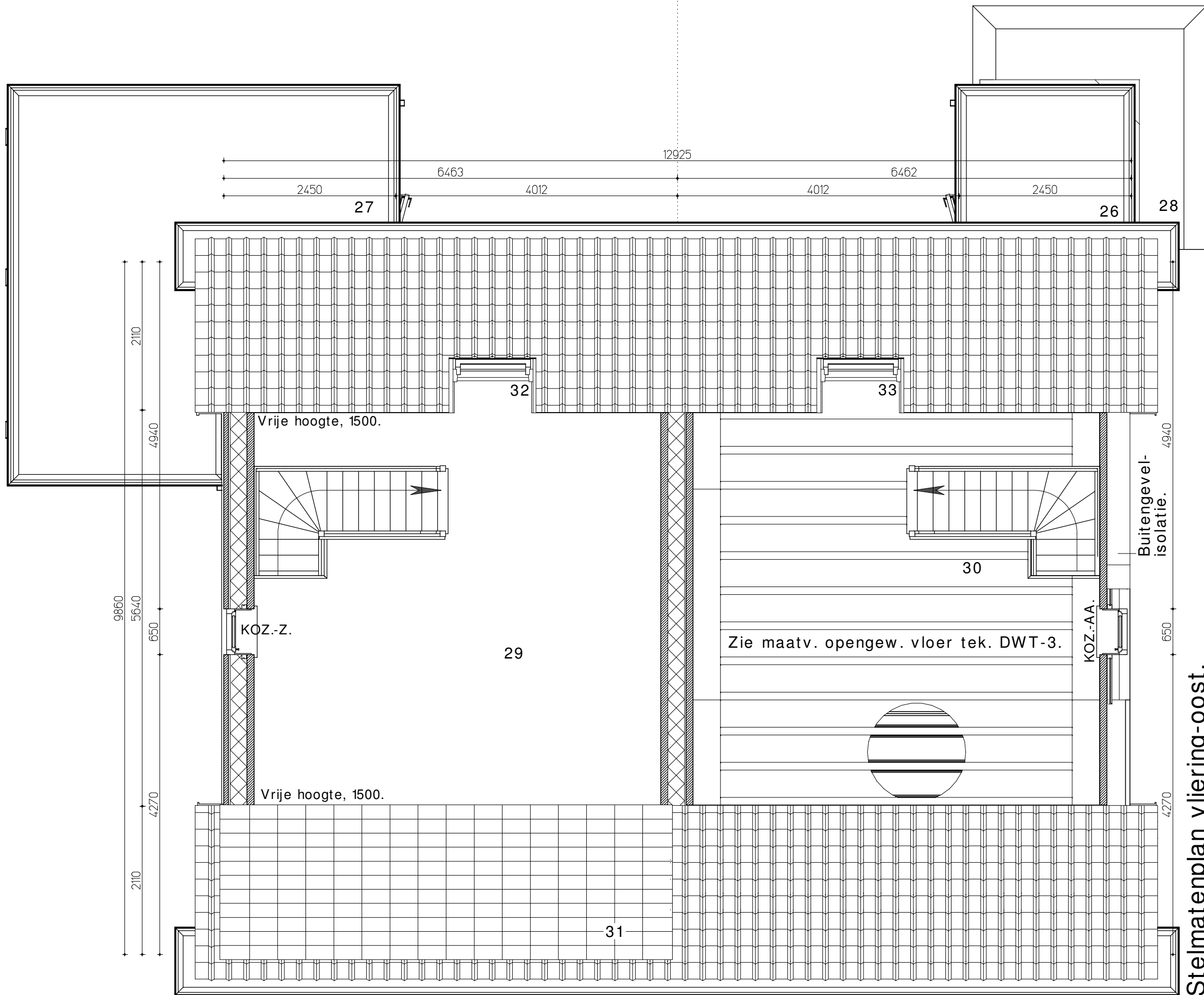
Stelmatenplan vliering-west.
